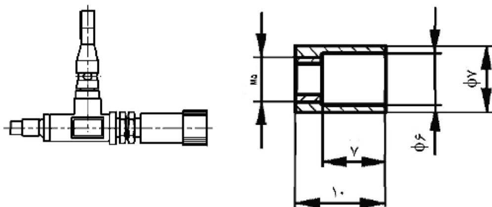
شکل 2-ج ( مشعل و شیر تنظیم
